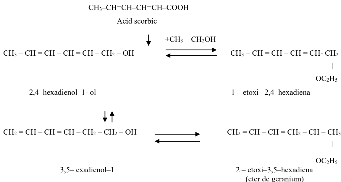
Fig. 1 – Mecanismul formării eterilor răspunzători de gustul dezagreabil de geraniu semnalat în urma metabolizării acidului sorbic de către bacteriile lactice (Edinger W. D. și Splittstoesser D. F., 1986a, 1986b; Rymon-Lipinski G. W. ș. a., 1975)
